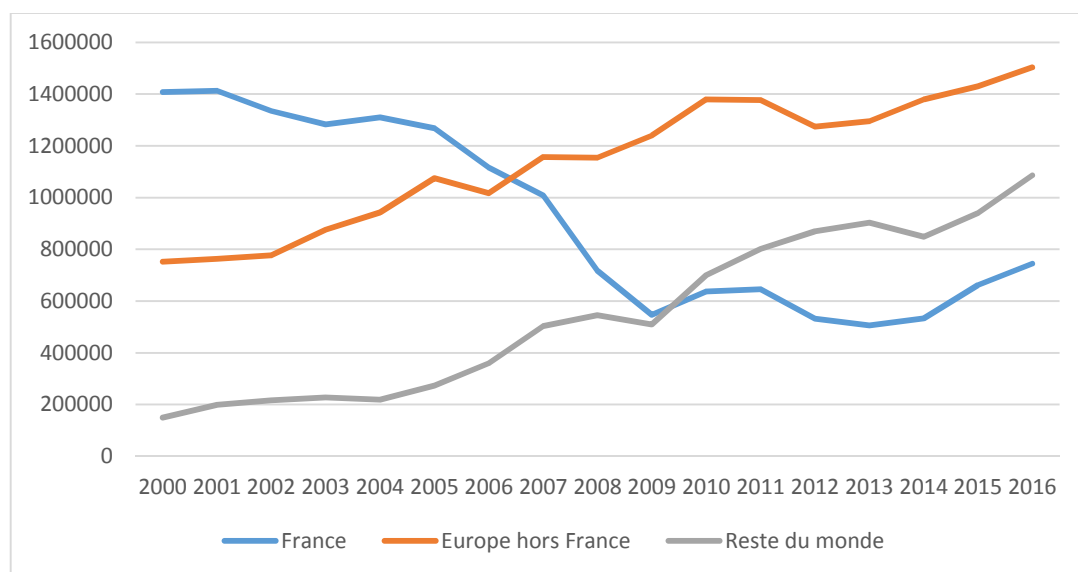
Graphique 20 : Production de Renault en France, en Europe (hors France) et dans le reste du monde (en nombre de VP et VU)
