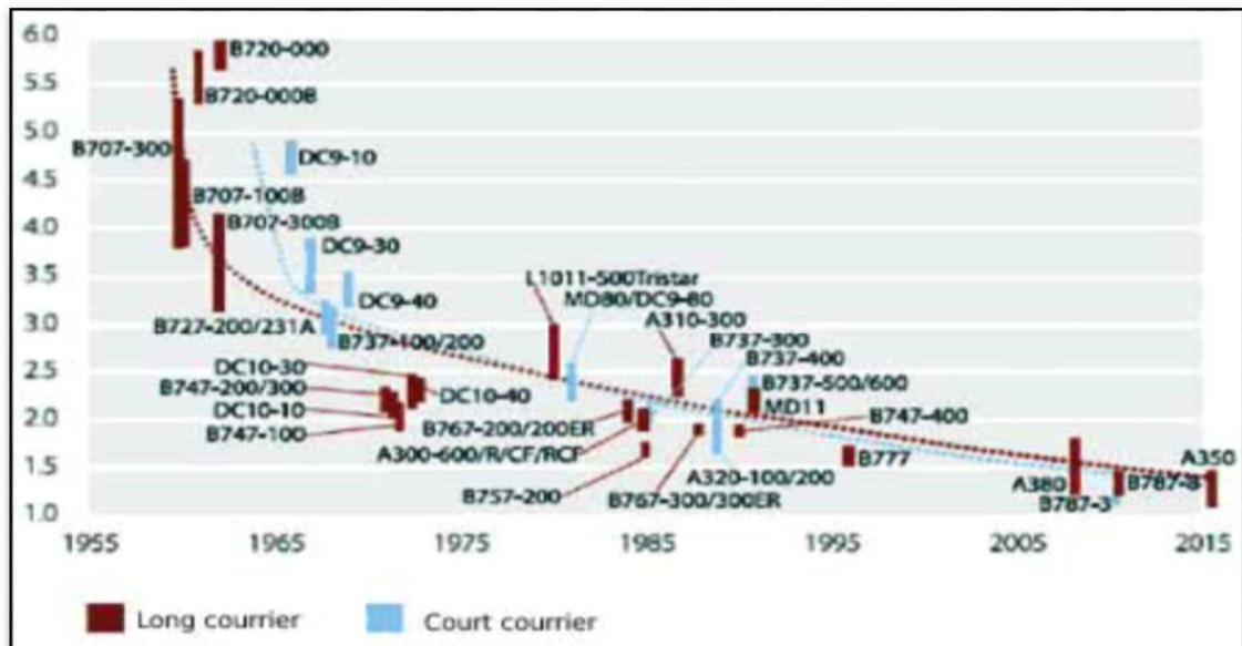
Graphique 25 : Efficacité énergétique (en mezza joule/km)
