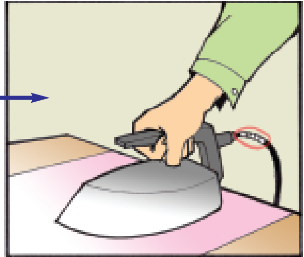
Hình 26: Hãy kiểm tra tất cả chỗ nối, cố định chúng bằng keo cách điện. Đừng để lại bất cứ chỗ nối nào mà không được bọc bảo vệ. Chắc chắn rằng không ai có thể chạm vào chúng.
