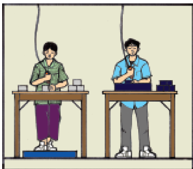
Hình 32: Sử dụng một bậc đứng cho người lao động có tầm vóc vừa và nhỏ, và bộ phận giữ đồ vật cho người lao động có thân hình cao để điều chỉnh chiều cao công việc của họ đến tầm khuỷu tay.
