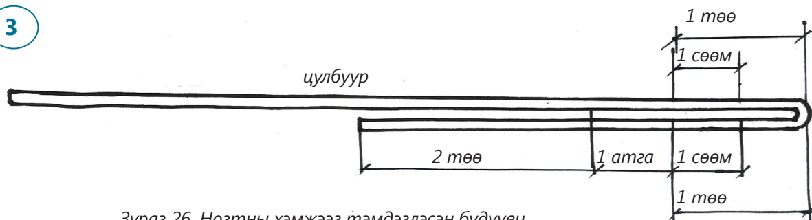
Зураг 26. Ногтны хэмжээг тэмдэглэсэн бүдүүвч
