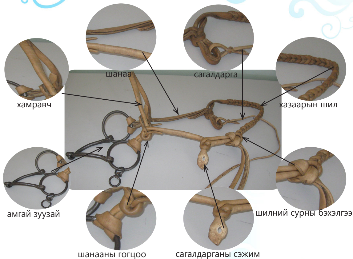
Зураг 24. Хазаарын бүрдэл хэсэг
