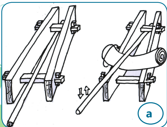
Зураг 12. а) банзан талхи, б) сур ээрүүлдэх хэрэгсэл
