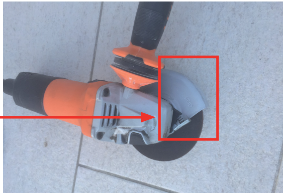
الصورة ٤٩. آلة قطع/جلخ يدوية مزودة بالحماية اللازمة.
