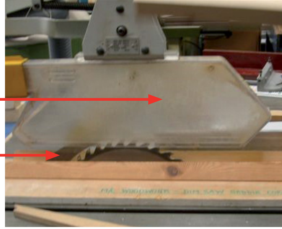
الصورة ٤٧. منشار دائري مزود بالواقي المناسب.
