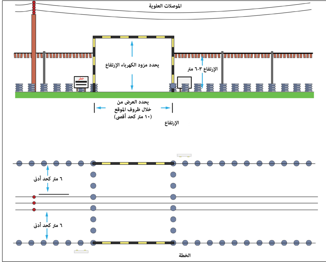
الصورة ٤٤. أمثلة عن الأبعاد المفروض مراعاتها لنقاط العبور والحواجز.
