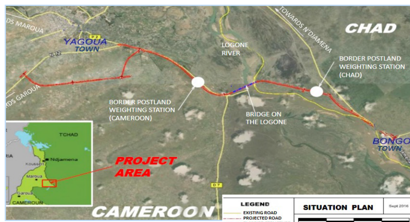
Carte de la zone du projet de construction du pont et de la route entre Yagoua (Cameroun) et Bongor (Tchad)
