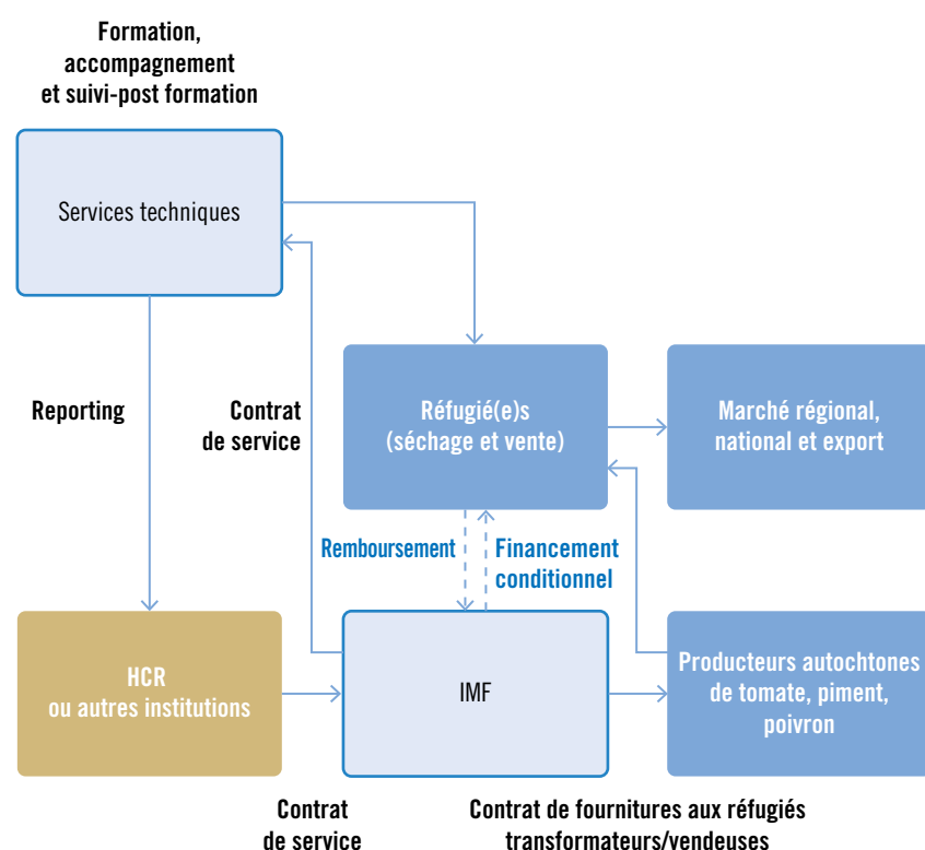
Figure 16: Opportunité d'intervention en séchage, stockage et commercialisation de produits maraîchers
